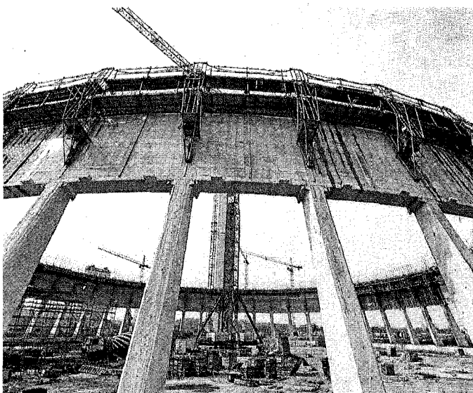
Auf der Baustelle des Trianel-Kraftwerkes wächst der Kühlturm in die Höhe.
