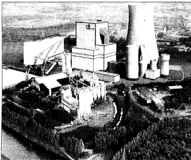
Wenn Arnberg die Genehmigung erteilt, will Trianel sein Steinkohlekraftwerk (hier im Modell) in Lünen bauen und nicht nach Krefeld „verschieben“. (Fotomontage: Archiv)
