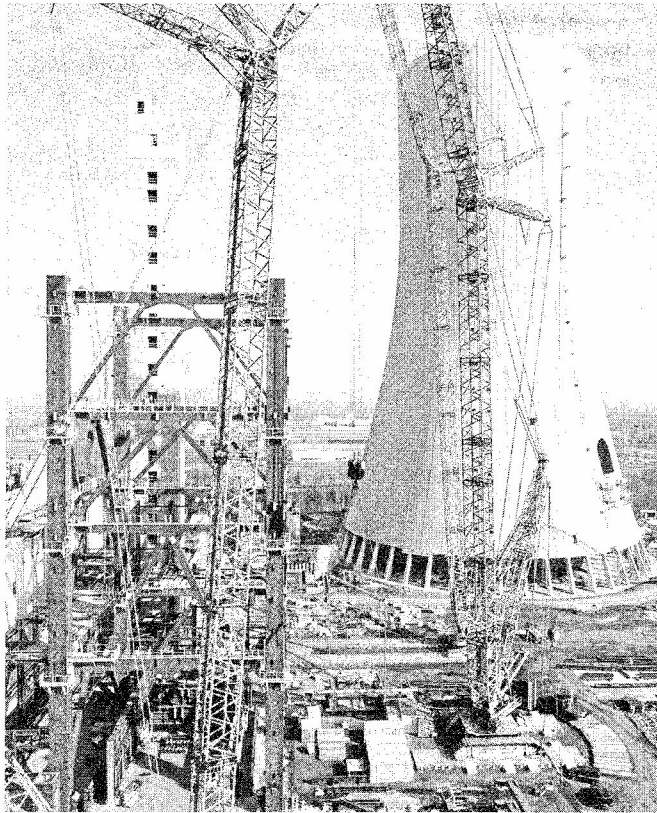
Die Baustelle des Trianel-Kraftwerks in Lünen.
