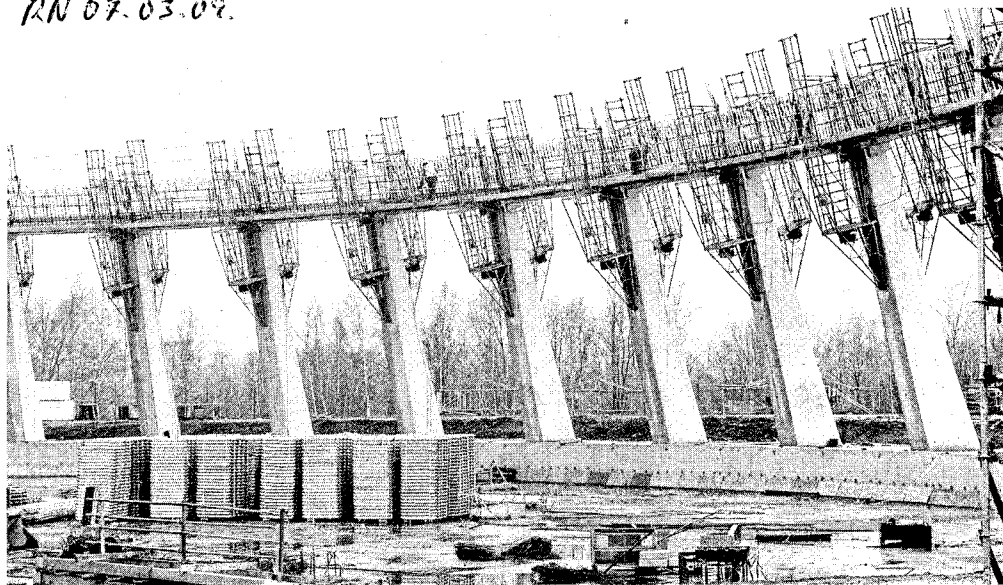
Auf der Baustelle des Kraftwerks wächst bereits der Kühlturm in die Höhe. Für Trianel steht fest: Wir bauen weiter..
