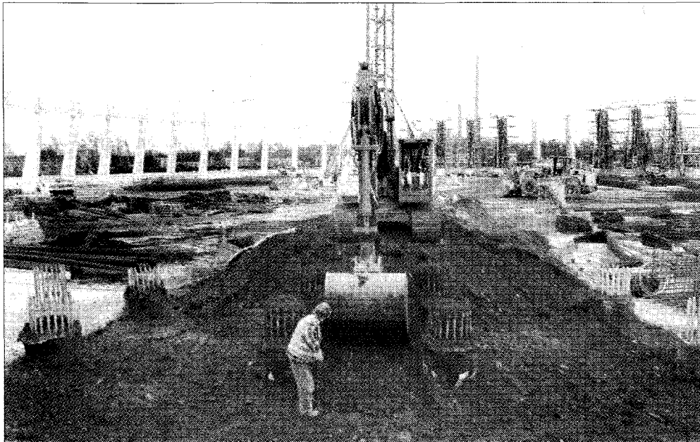
Der Kraftwerksbau – hier die Arbeiten für den Kühlturm – liegt nach Angaben von Trianel im Zeitplan, obwohl die Baustelle im Januar eine Woche stillgelegen hat. (Foto: Günter Blaszczyk)
